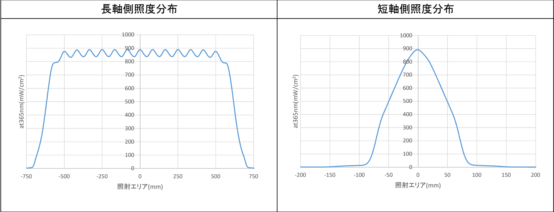
照度分布(代表例 照射エリア長軸1000mm)
