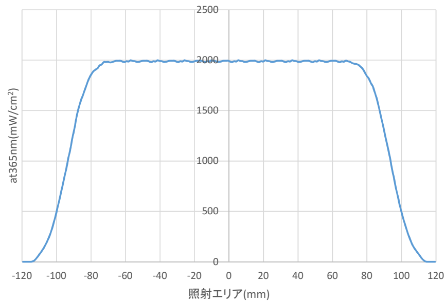
長軸側照度分布
