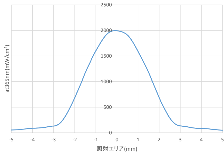
短軸側照度分布
